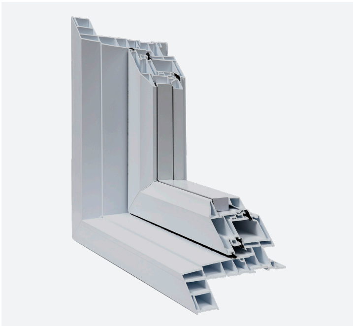
CADRE + MOULURE À BRIQUE STYLE TRADITIONNEL ½" et 1"
