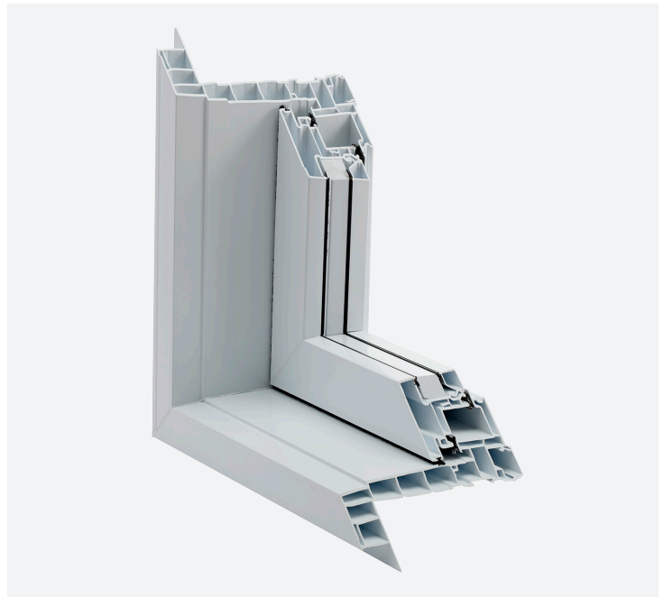
CADRE + MOULURE À BRIQUE STYLE CONTEMPORAIN ½" et 1"
